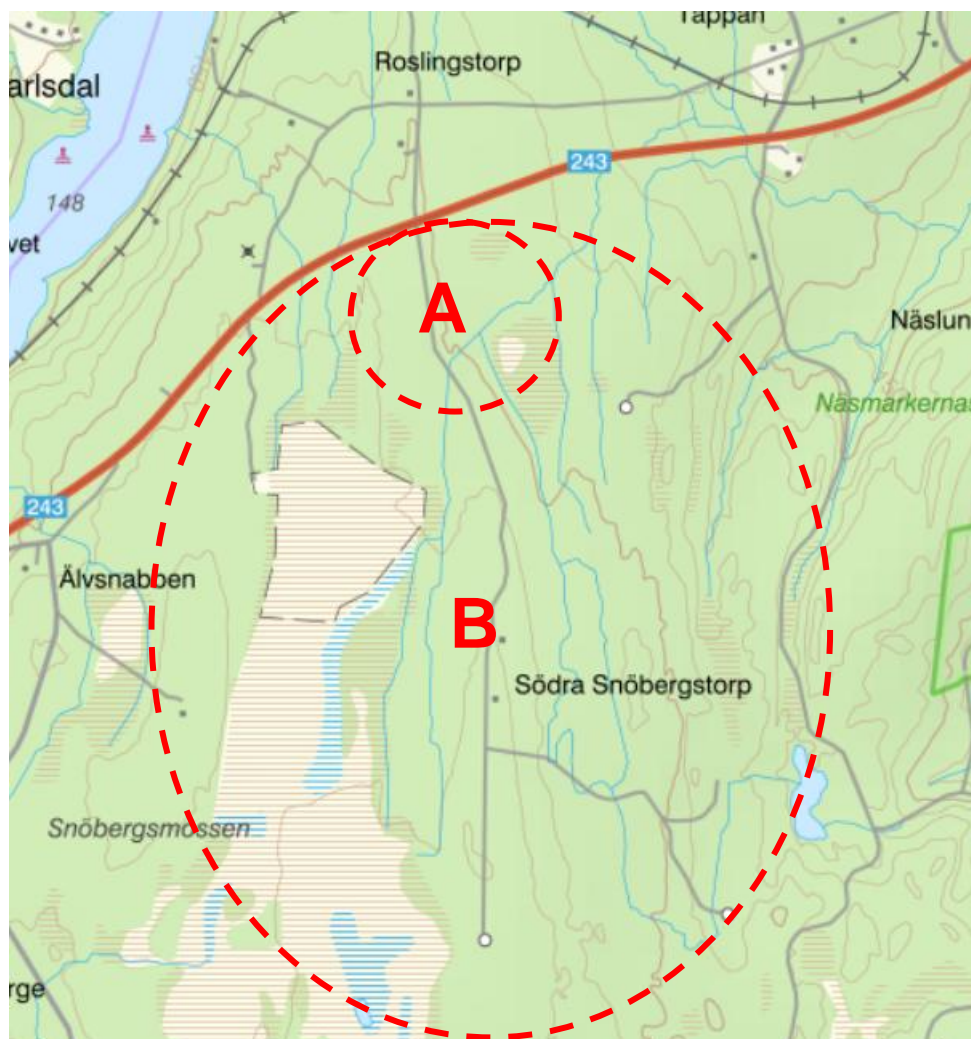
Figur 1 Dunderberget: Grov kartbild över ungefärligt område. Observera att områdena är grovt uppskattade och har stort utrymme för manövernåm beroende på hur man väljer att placera anläggningarna. Säkerhetsavstånd A: cirka 430 meter. Säkerhetsavstånd B: cirka 1240 m.
