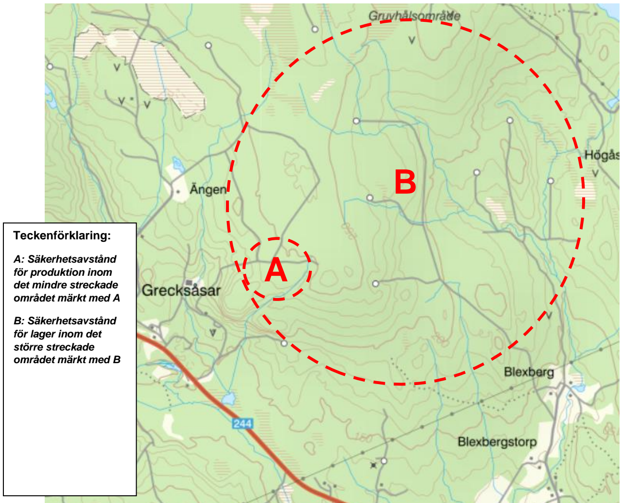
Figur 4 Grecksåsar: Grov kartbild över ungefärligt område. Observera att områdena är grovt uppskattade och har stort utrymme för manövern beroende på hur man väljer att placera anläggningarna. Säkerhetsavstånd A: cirka 430 meter. Säkerhetsavstånd B: cirka 1240 m
